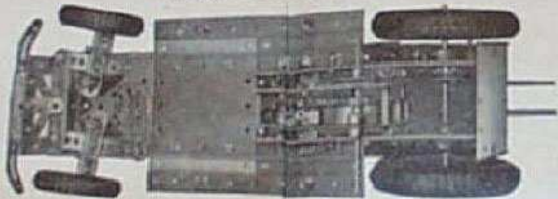
Abb. 52.8a Unteransicht des Kronautos
