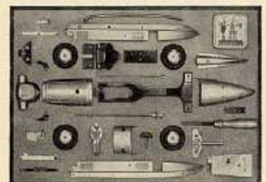
Rennauto, zerlegt, in Karton, mit Motor und Fahrer und ausführlicher Bau-Anleitung. No. 1133 Al — Aluminiumfarbig. No. 1133 R — Rot
