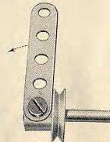
Nr. 10 Lose Verbindung mit Band und Schnurlaufrad
