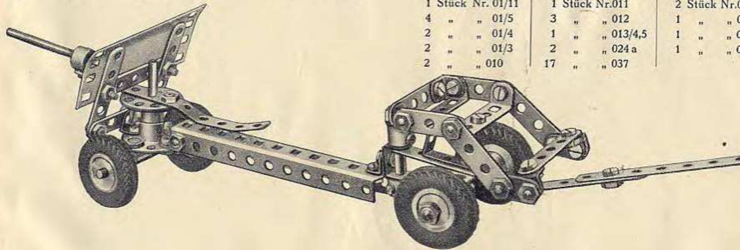
Nr. 01-50 Feldhaubitze mit Protze
