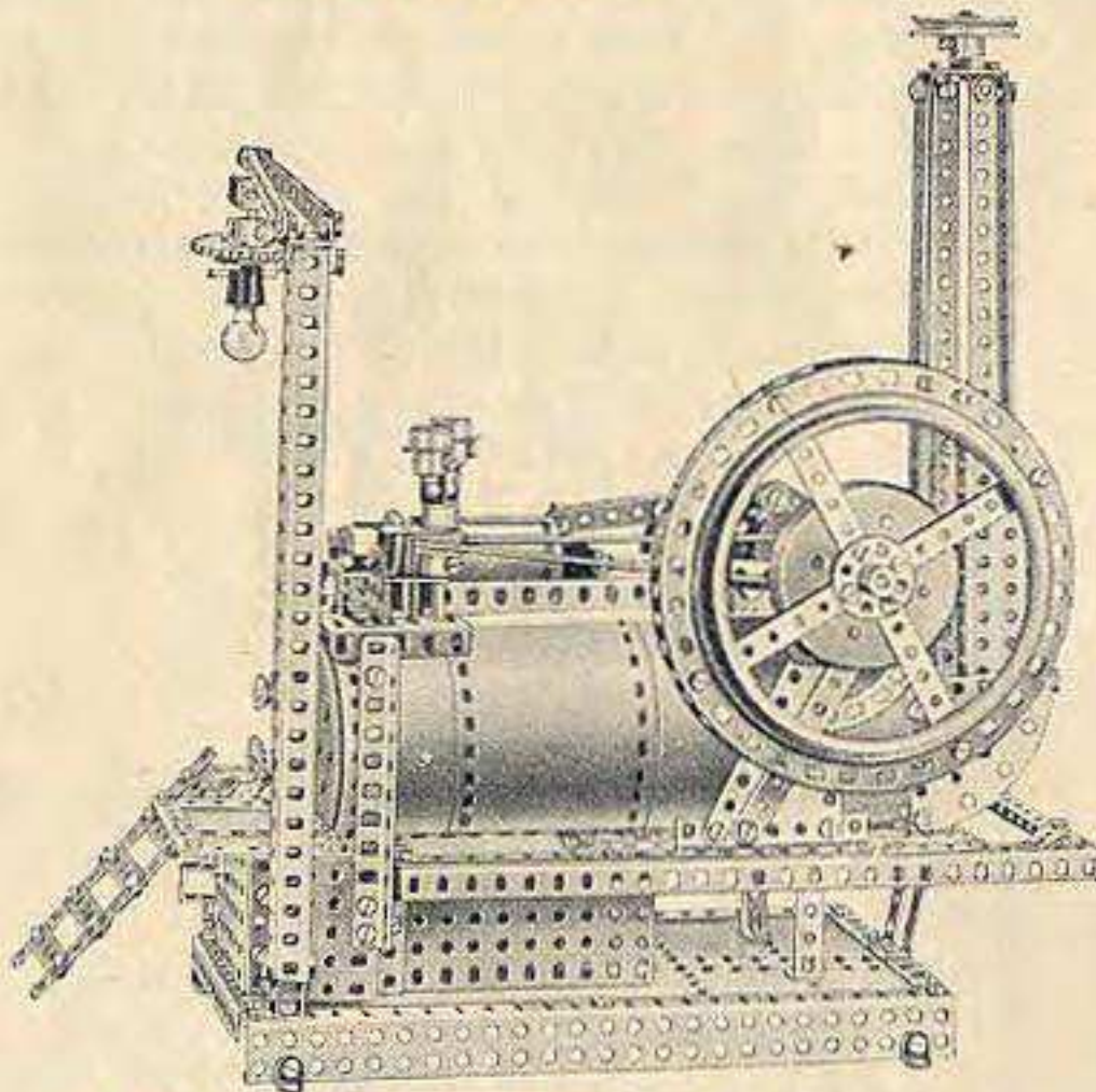
Lokomobile mit Unterbrechermotor (gebaut mit Kasten 03)
