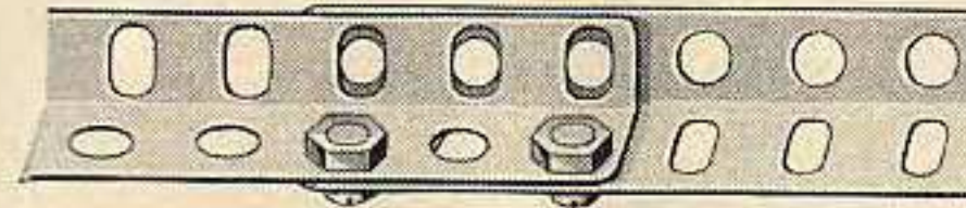
Nr. 3 Überlappung zweier Winkelträger
