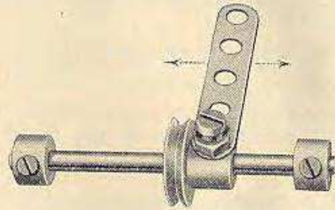
Nr. 11 Führung mit Band und Welle
