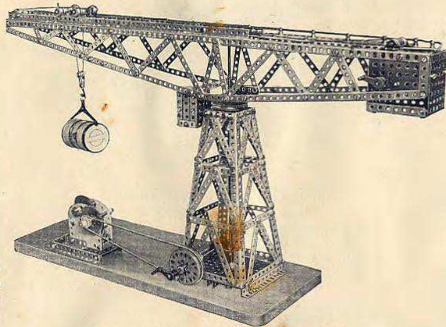
Hammerkran mit Elektromotor 0301 (gebaut mit Kasten 03)
