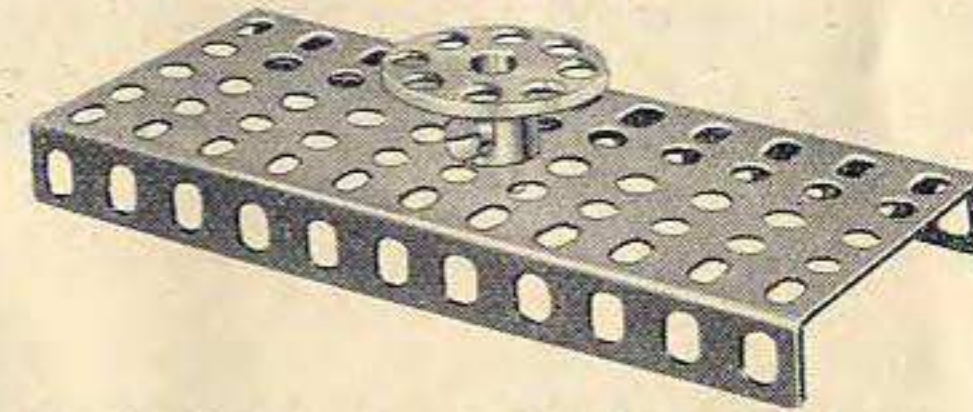
Nr. 16 Schraube als Zapfen auf Platte
