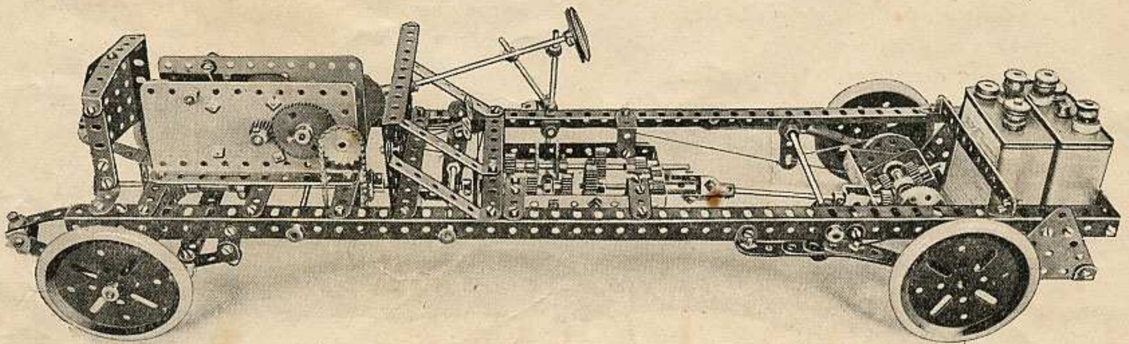
Châssis automobile
