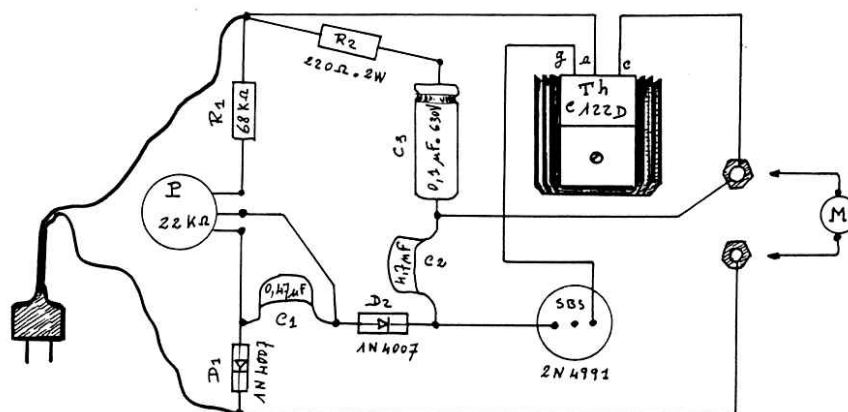
Schema de Câblage
