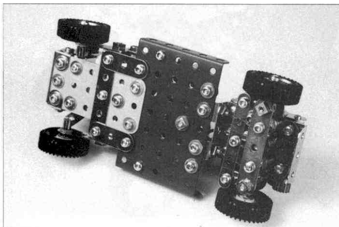
Fig. 5 : La plate-forme technique vue de dessous. La composition en 3 parties apparaît clairement.
