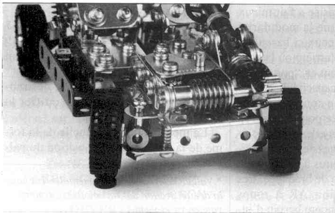
Fig. 9 : La suspension AV droite est comprimée par le passage de la roue sur un obstacle. Noter le mouvement "vertical" de l'ensemble roue, pivot de roue et biellette de direction.
