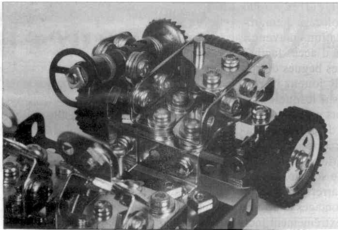
Fig. 7 : Le berceau AV vu de 3/4 AR. Le pignon de 19 dents et la vis sans fin sont fermement maintenus pour un engrènement mutuel correct.
