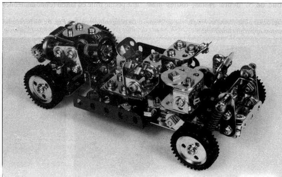
Fig. 2 : La plate-forme technique. Remarquer l'emploi de pièces de création récente pour représenter les sièges et la suspension AR.
