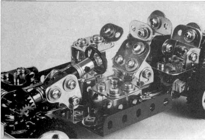
Fig. 3 : Le plancher central. On distingue les systèmes de guidage longitudinal des sièges et d'inclinaison des dossiers. Le petit volant est une pièce Meccano.
