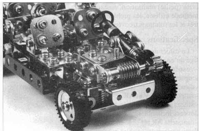
Fig. 6 : Le berceau AV, regroupant direction et suspension. Le pignon de 15 dents a été retenu pour un encombrement réduit.
