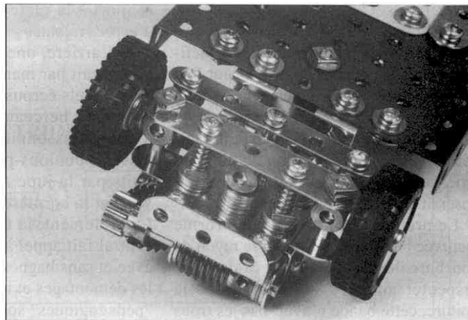
Fig. 8 : La direction et la suspension AV. La bande normale de 5 trous assure à elle seule la "triangulation" inférieure droite et gauche. La bande étroite est flottante.
