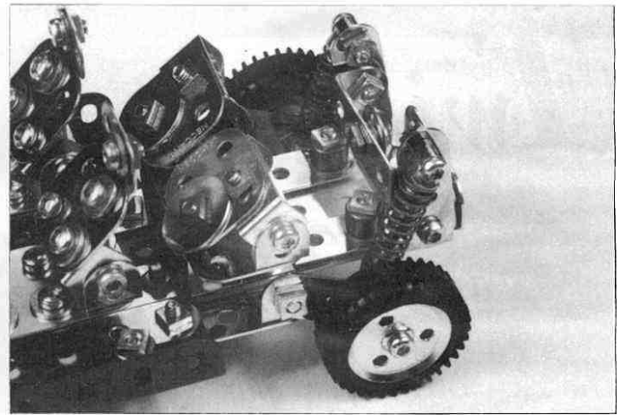
Fig. 4 : Le berceau AR. Les demi-dossiers de la banquette sont rabattus. Les bras tirés de la suspension AR sont des bandes de 3 trous.
