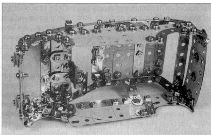
Fig. 10 : L'intérieur de la carrosserie montre les nombreux renforts utilisés pour rigidifier la coque. Remarquer l'emploi de rares équerres et supports plats étroits non fabriqués par Meccano.
