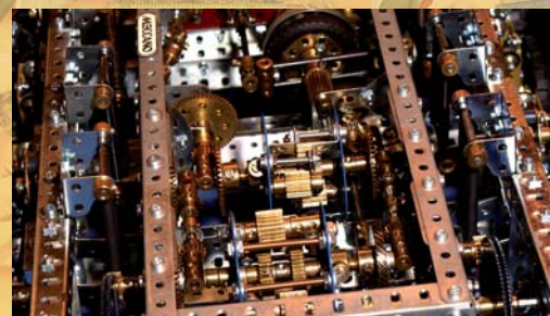
Châssis à chenilles à transmission Gleasman de Michel Perrin
