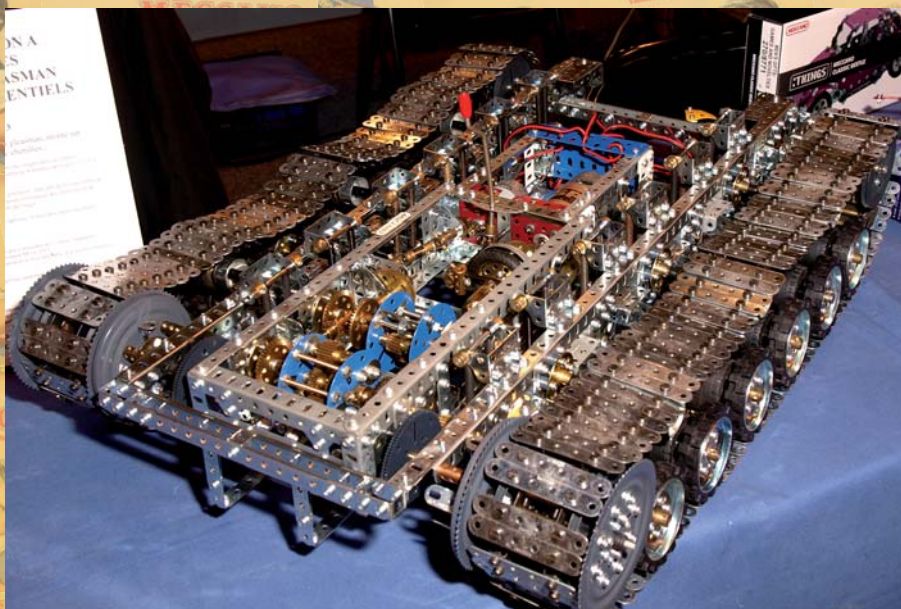
Châssis à chenilles à transmission Gleasman de Michel Perrin
