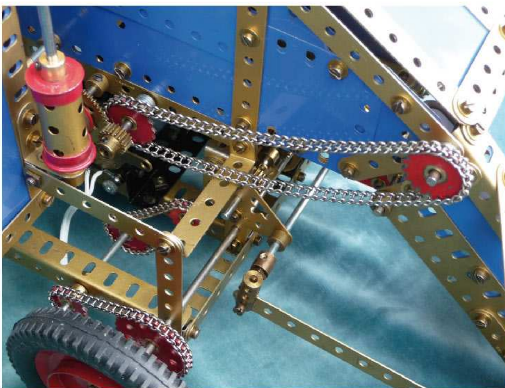
Transmission du mouvement
