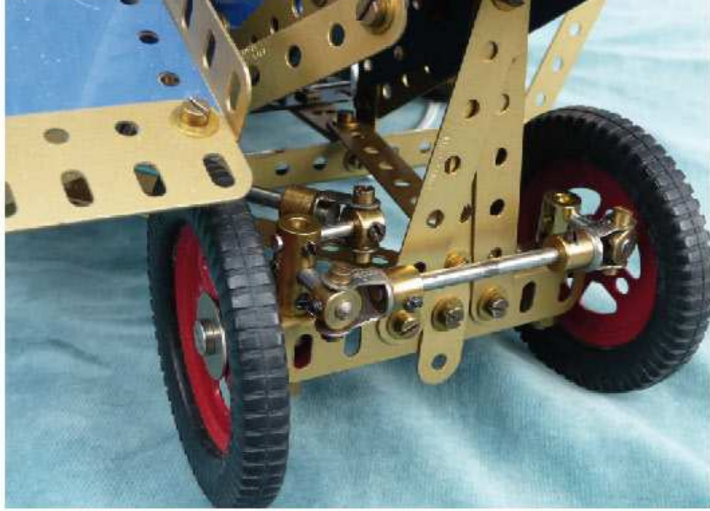
Mécanisme d'orientation des roues
