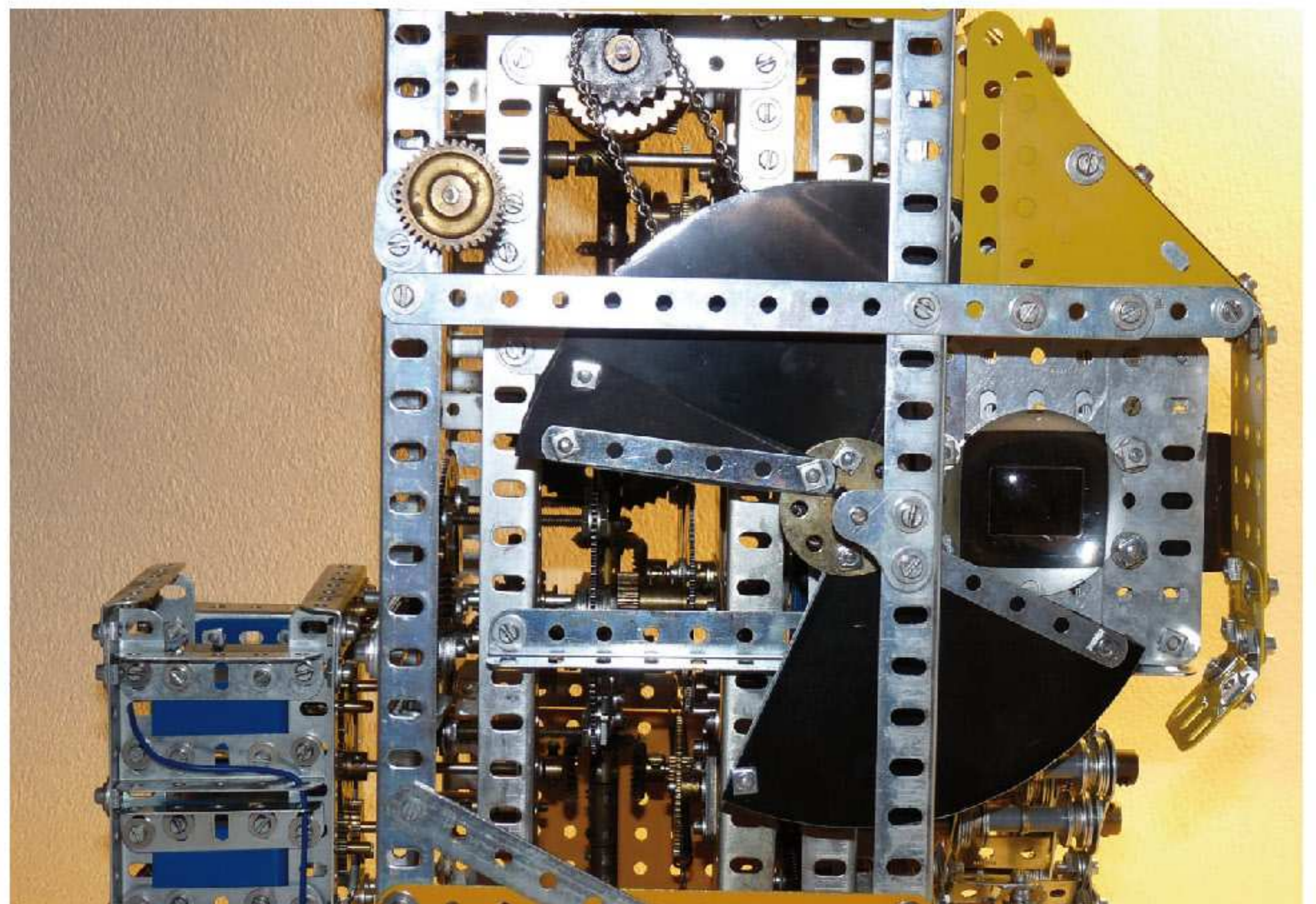
La face arrière du mécanisme avec l'obturateur et la fenêtre de projection
