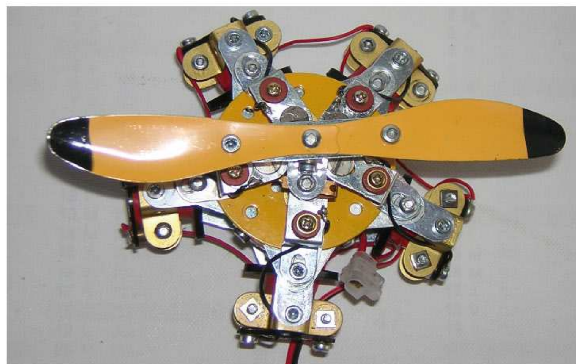
Moteur en étoile 5 cylindres de Willy Dewulf Ces constructions sont inspirées d'anciens Meccano Magazine. Contrairement au moteur 6 cylindres en ligne d'Aubin Fanard (voir CAM N° 100), l'ordre d'allumage de ces moteurs est circulaire au lieu de respecter celui des véritables moteurs : 1-3-5-2-4 pour l'étoile et 1-5-3-6-2-4 pour le moteur en ligne.
