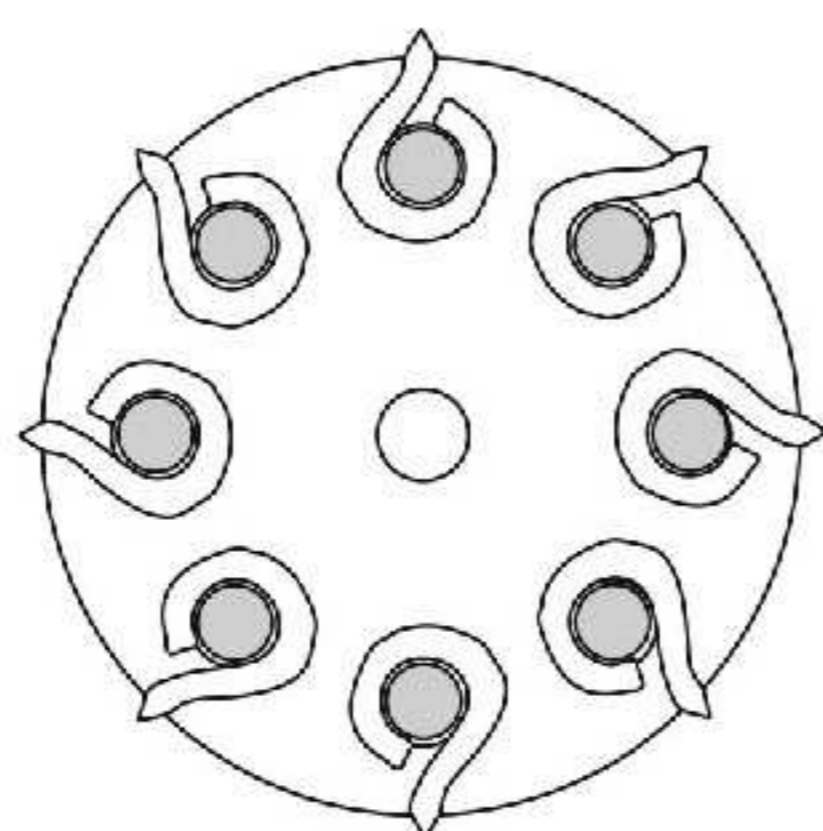
Solution retenue pour l'entraînement du film
