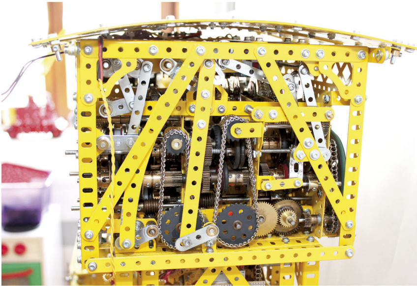
Fig. 13 Vue de la partie transmission depuis la face arrière
