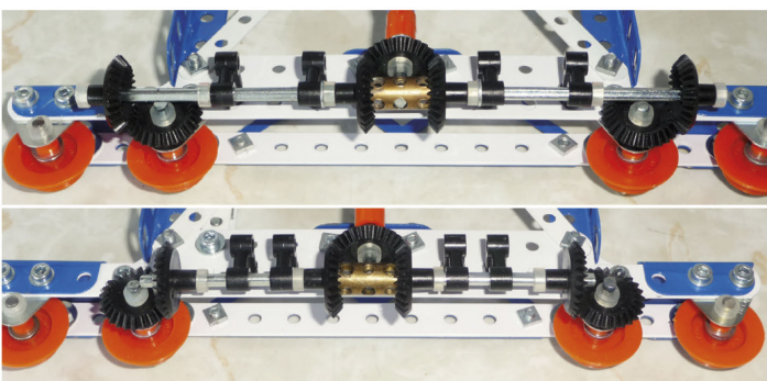
Fig. 8 Les entraînements des roues
