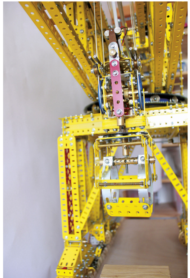
Fig. 15 La pince avec le pendule (bande 6 trous rouge) utilisé pour la mise à niveau automatique de la pince (correcteur d'assiette)
