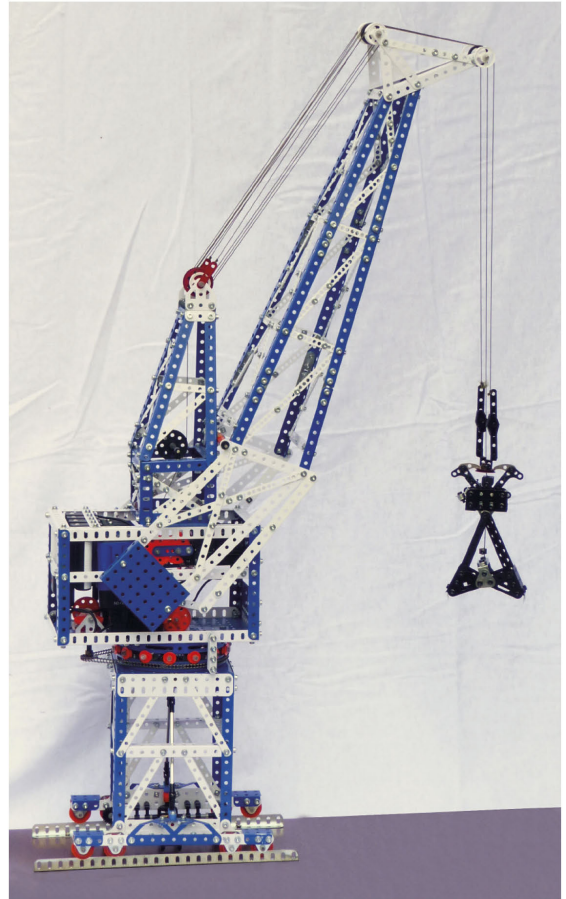
Fig. 5 La mini SM35
