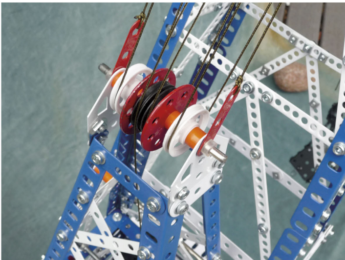
Fig. 22 Les poulies en tête de tour
