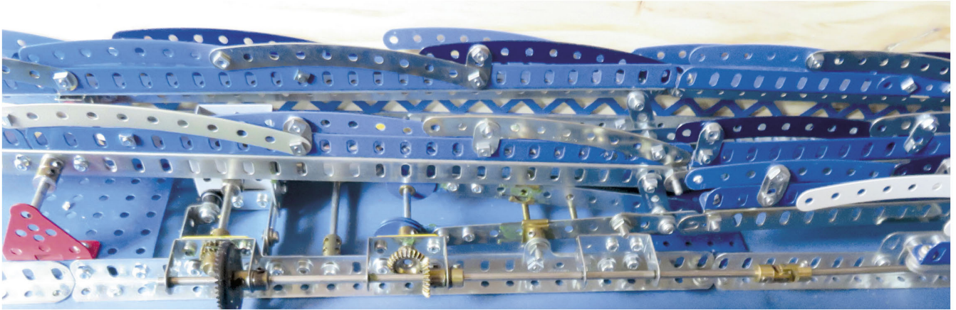
Fig. 6 Le mécanisme des vagues de devant constitué de chaque coté par un excentrique relié à un bout de l'élément central (celui de la dernière vague est enlevé)
