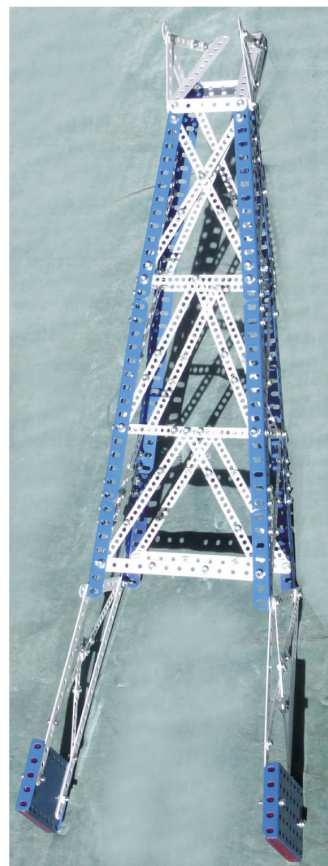
Fig. 14 La flèche, vue de dessus
