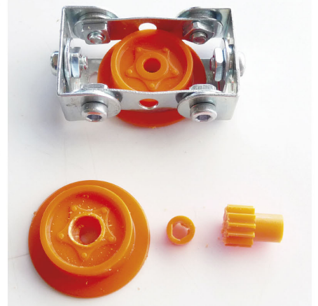
Fig. 30 Modification d'une roue à boudin
