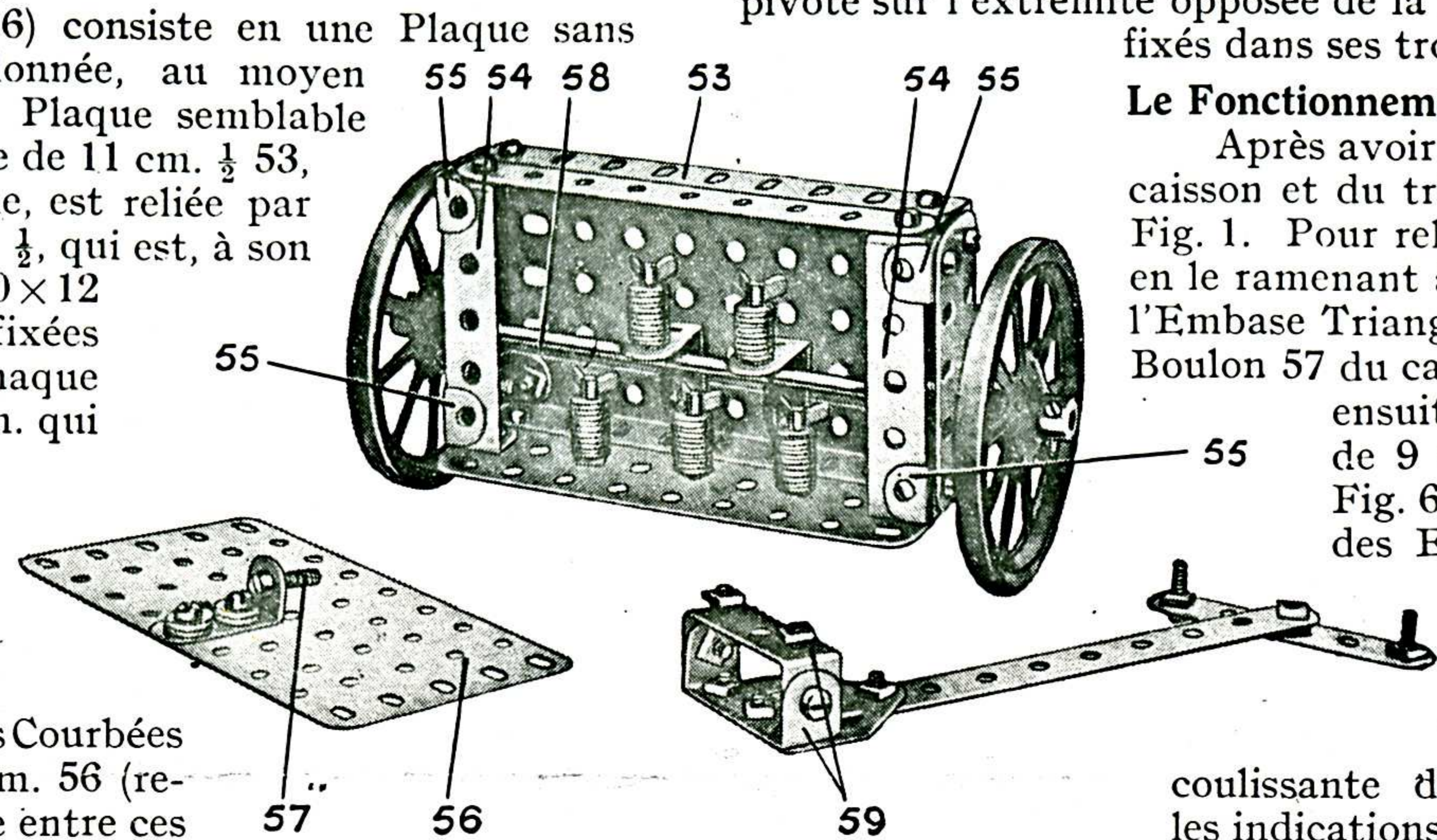
Fig. 6 Le caisson du modèle chargé de Rondelles-projectiles. La Plaque coulissante et la barre d'attelage sont représentées séparément.
