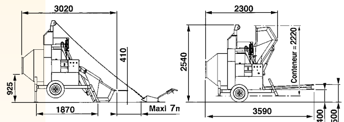
Accessoire : treuil pour chargeur
