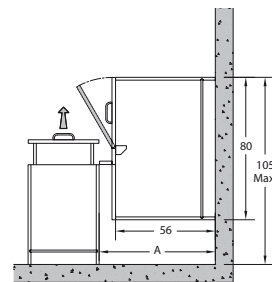
Meuble bas angle retour A = maxi 65 cm
