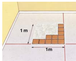
Départ de la pose
