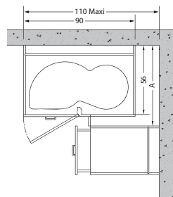
Meuble bas Nuoola A = maxi 65 cm
