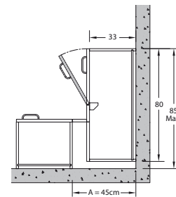
Meuble haut angle droit 90°
