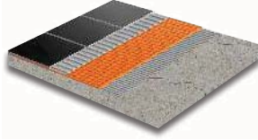
Carreler sur un sol fissuré (fissures inférieures à 2 mm)
