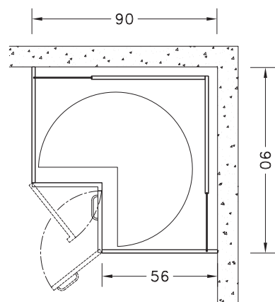
Ouverture droite. Meuble bas à 90° 2 portes avec fileur assorti
