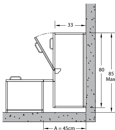
Ouverture droite. Meuble haut angle droit 90° A = mini 37 cm - maxi 45 cm
