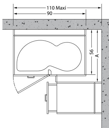
Ouverture droite. Meuble bas Nuvola A = mini 60 cm - maxi 65 cm
