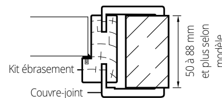
Porte + kit ébrasement (ou kit chambranle/contre-chambranle) pose en fin de chantier
