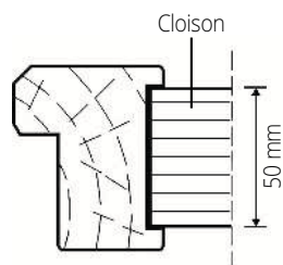
Huissier 67 ou 68 mm pour cloison de 50 mm
