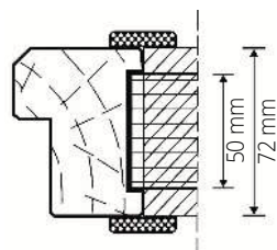
Huissier 72 mm pour cloison de 50 mm ou 72 mm (couvre-joint supplémentaire)
