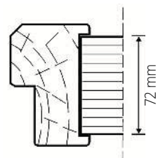
Huissier 88 à 92 mm pour cloison de 72 mm
