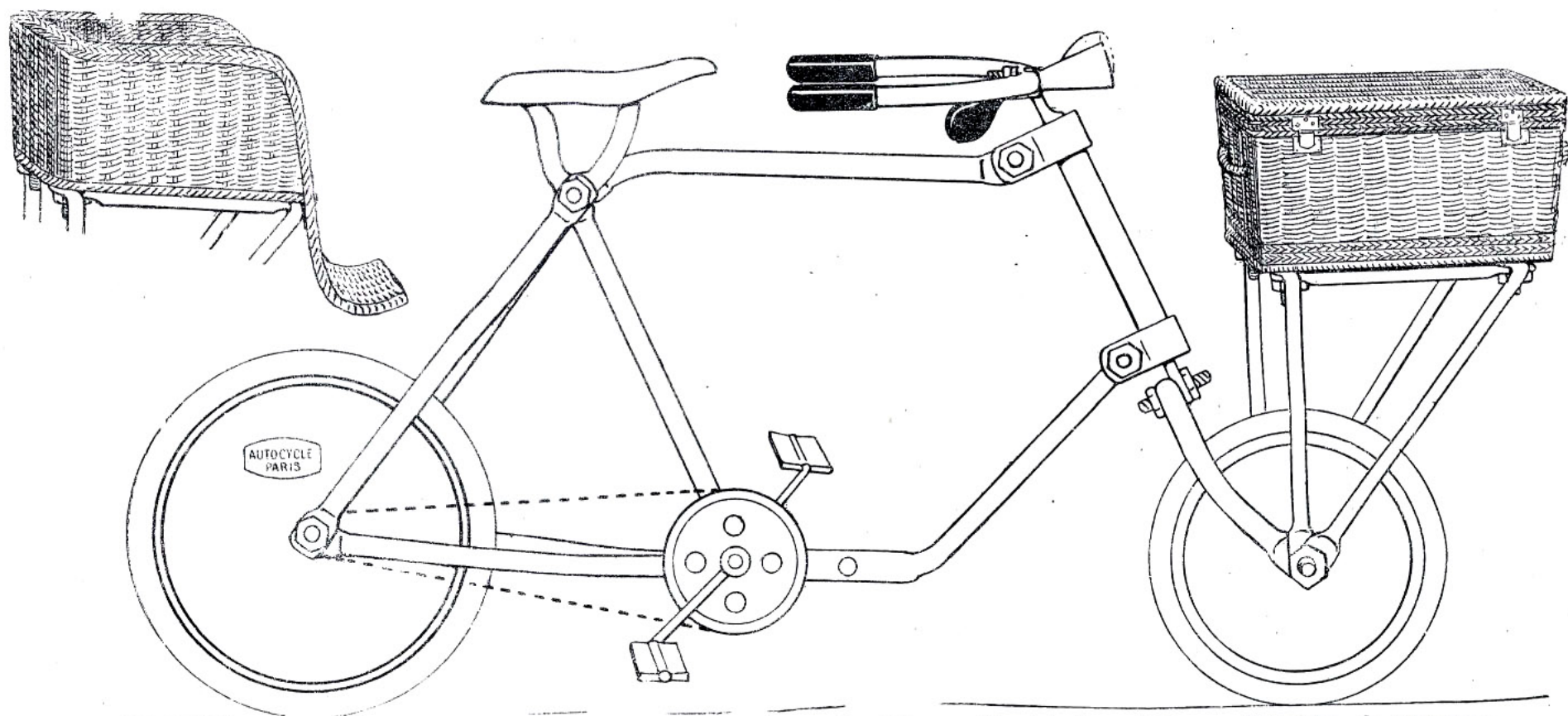
Bicyclette de Livraison
