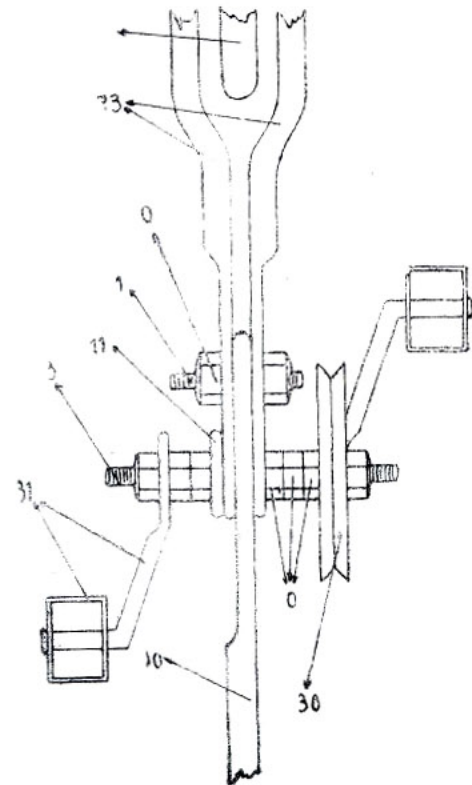
Motor falso Quicio do tri portador Pedal
