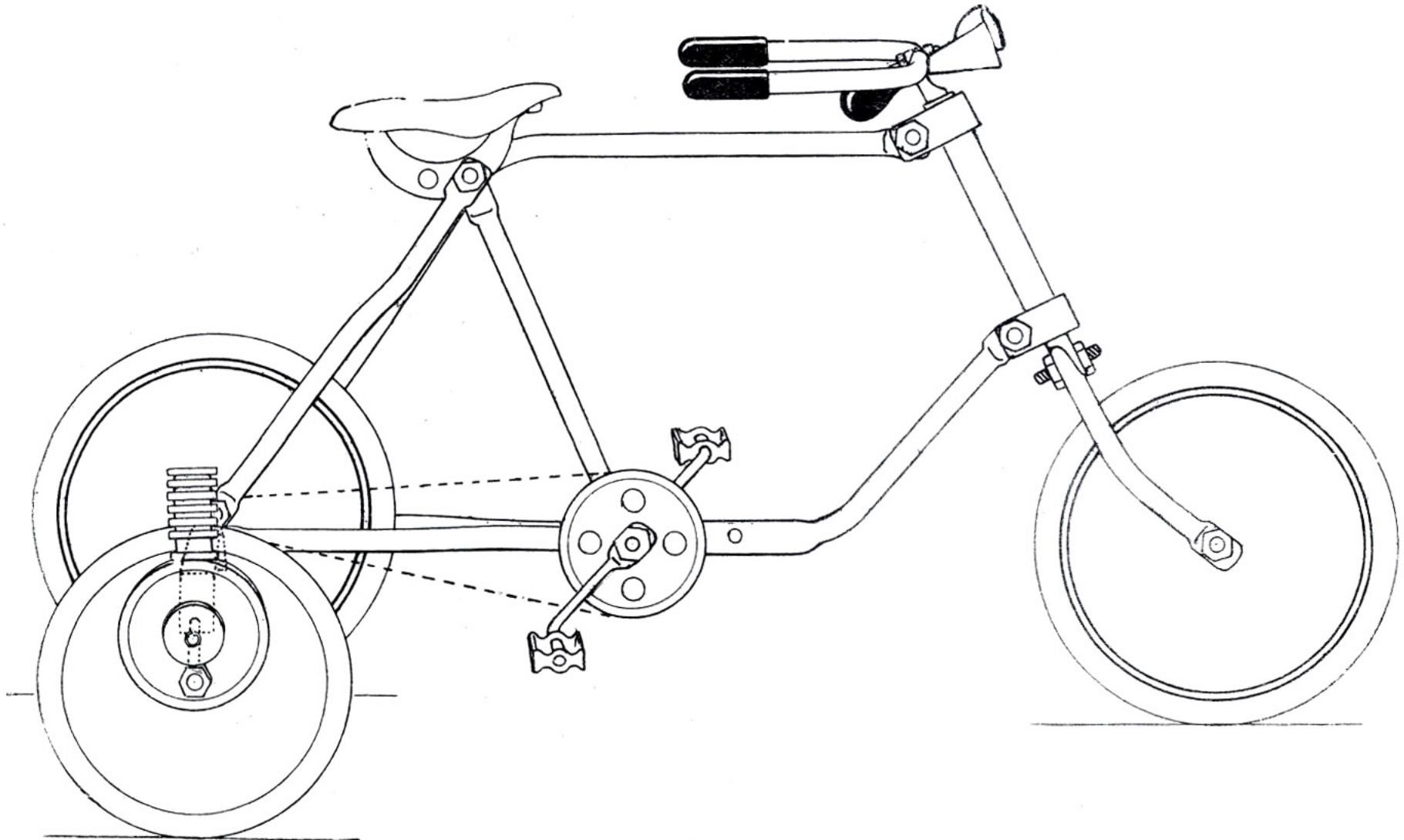
Bicyclette à roue auto
