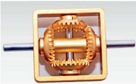
BG02 | Differential einfach
