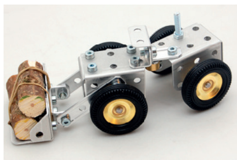
SN87 | Mini Bulldozer Schaufel, Räder, Gelenk beweglich (ohne Holz)
