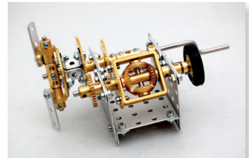
BG11 | Überlagerungsgetriebe
