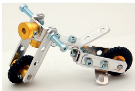
SN80 | Mini Töff Lenkung und Räder drehbar
