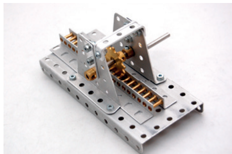
BG14 | Zahnstangengetriebe
