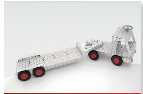
SN03 | Lastwagen 2-Achser mit 2-achsigem Tieflader
