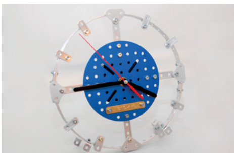
SN41 | Quarz-Uhr mit Uhrwerk
