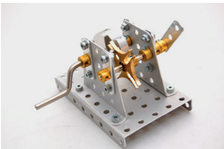
BG13 | Schrittschaltgetriebe
