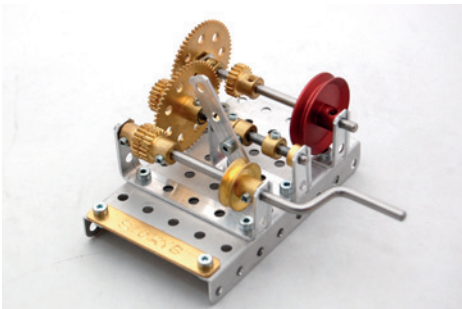
BG06 | Schaltgetriebe
