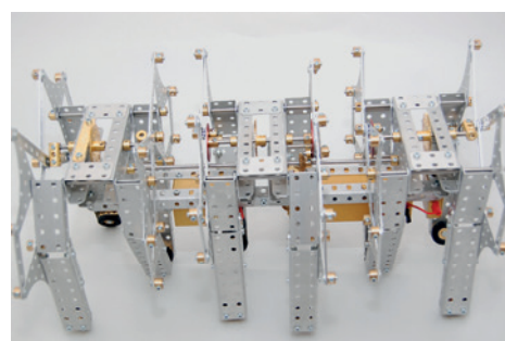
SE50 | Shongololo 12-Füssler
