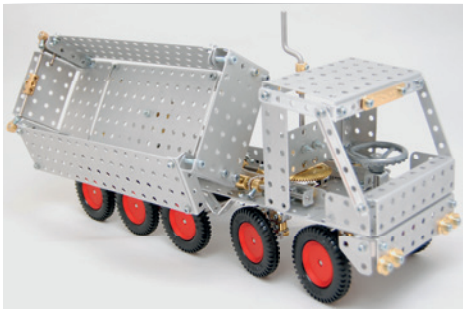
SN23 | Lastwagen 5-Achser Duo-Lenkung als 3-Seiten-Kipper
