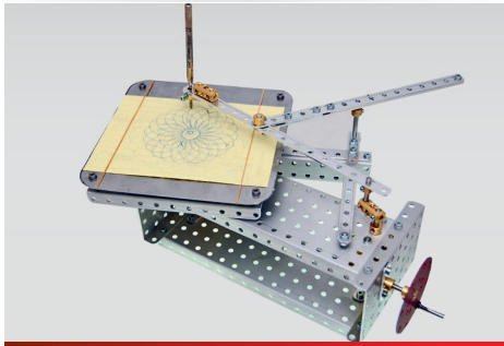
SN06 | Zeichnungsmaschine
