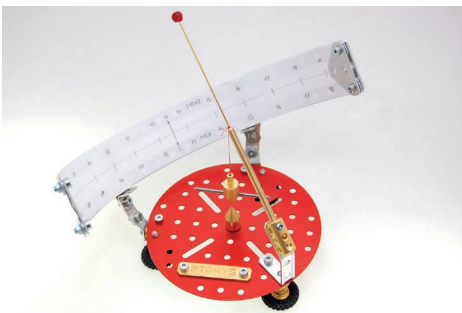
S011/S012 | Sonnenuhr
