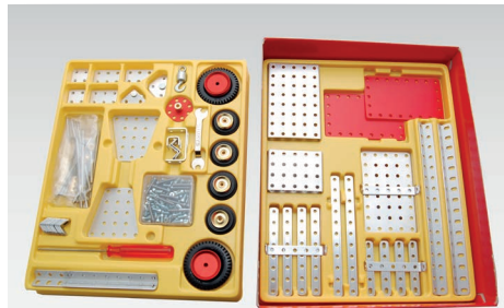
GK01 | Grundkasten 1
