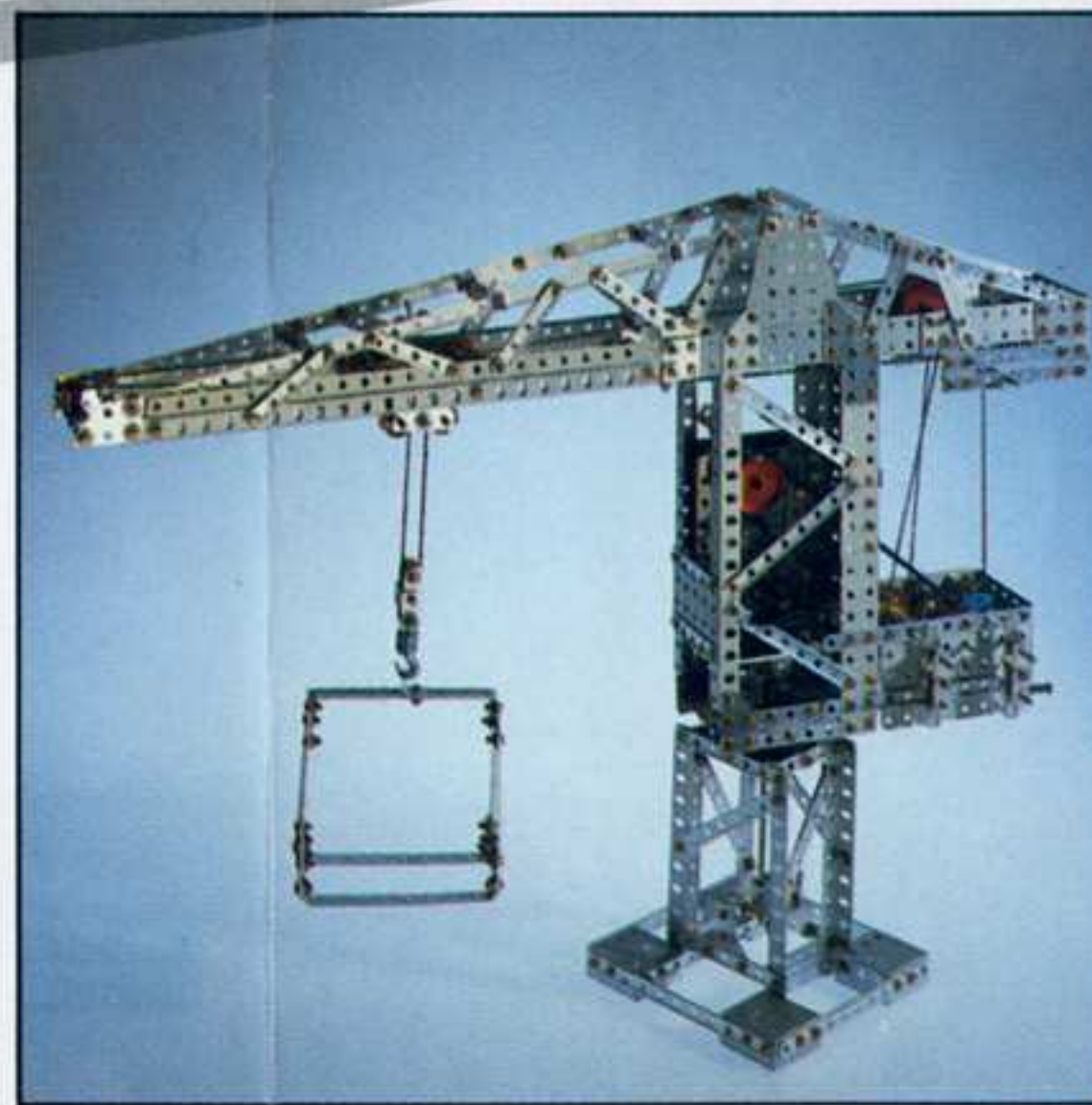
Grue à tour pivotante construite avec la boîte de base 3, entraînement par moteur à ressort.
