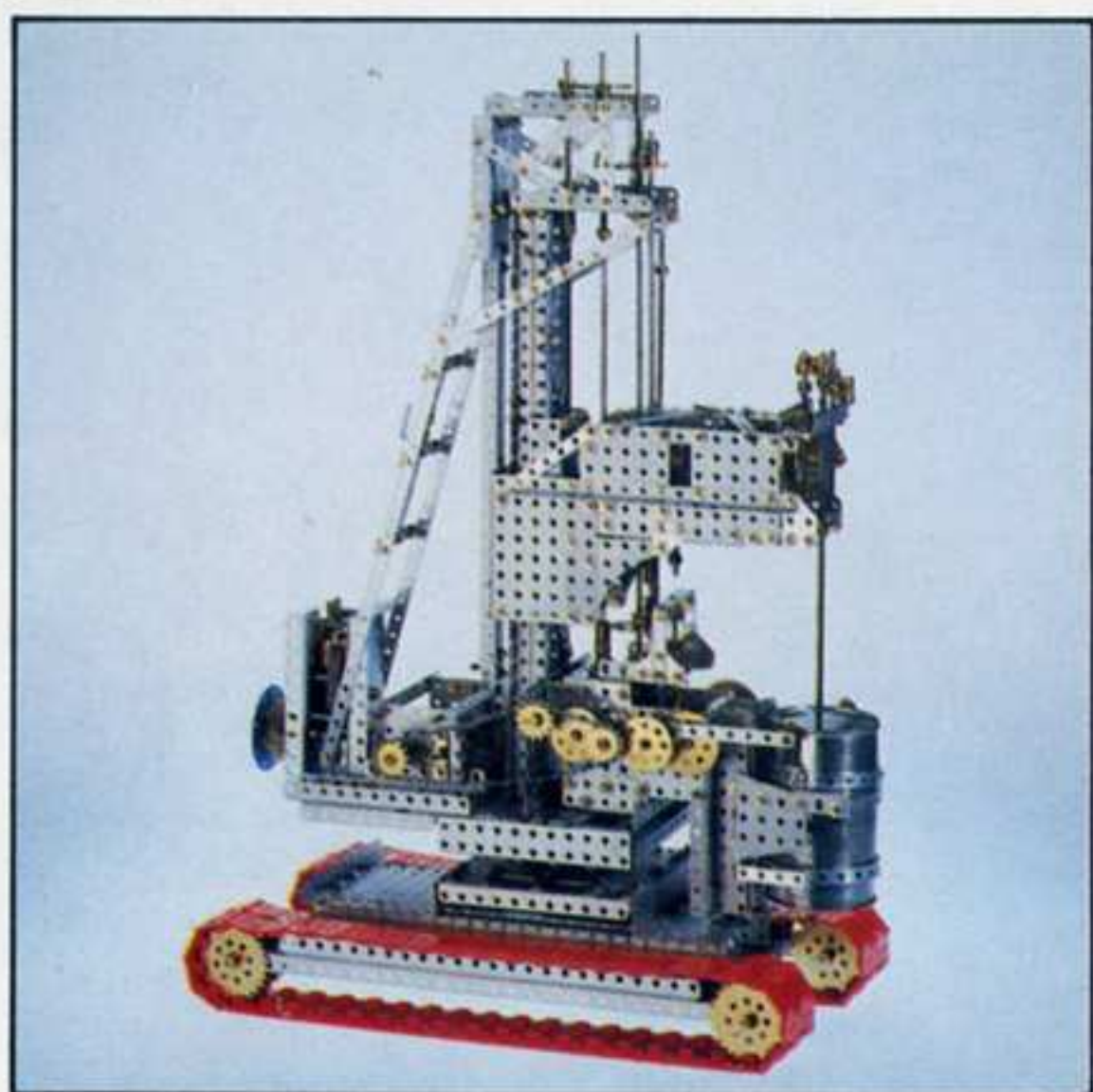
Batteuse de pieux construite avec les boîtes de base 4, G2 et pièces vendues au détail.
