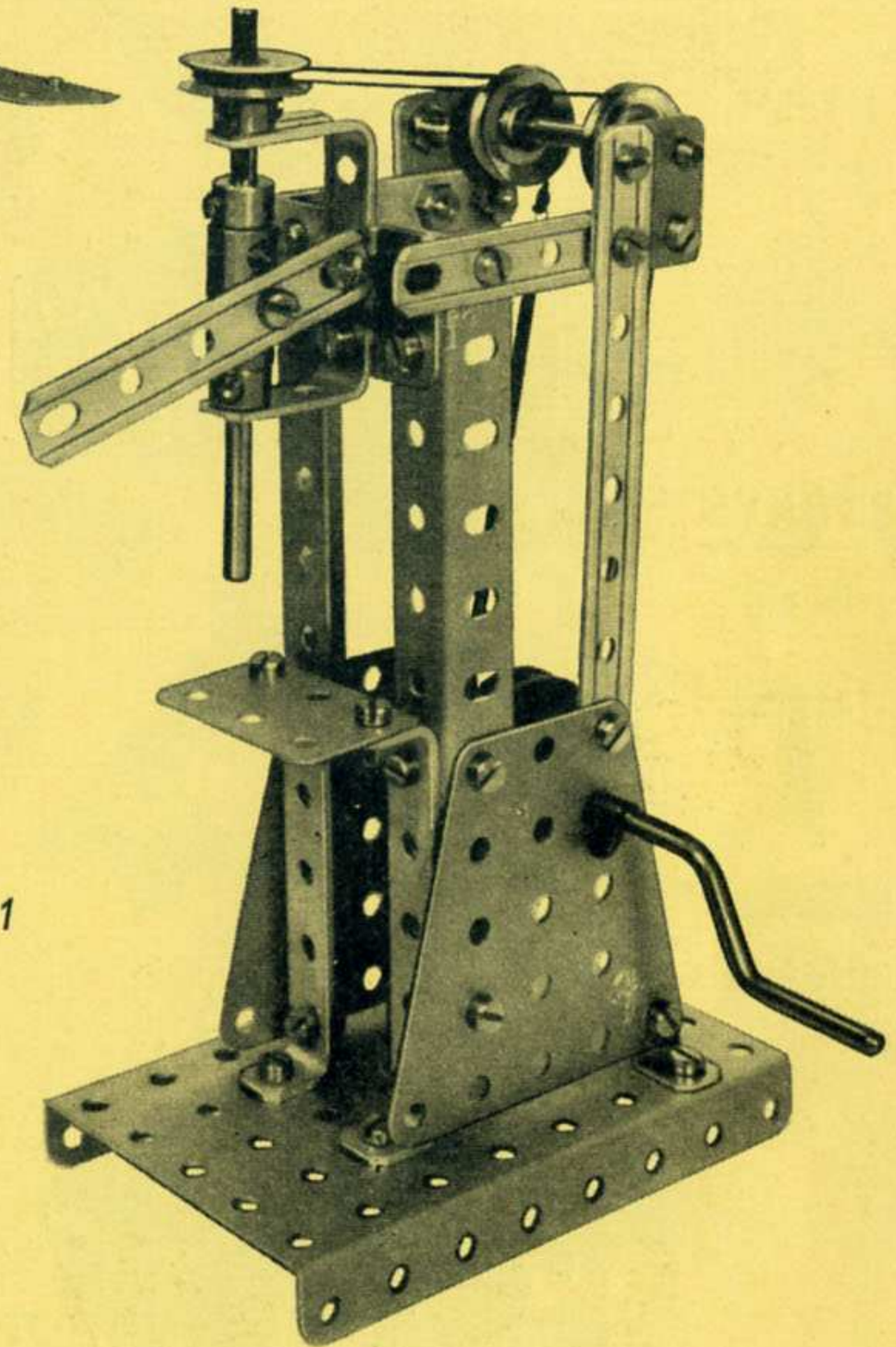
Gebaut mit Kasten 0 Construit avec boîte 0 Constructed with box no. 0
